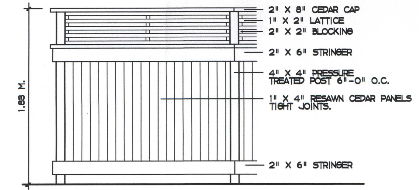
FENCE DETAIL SCALE: N.T.S.
